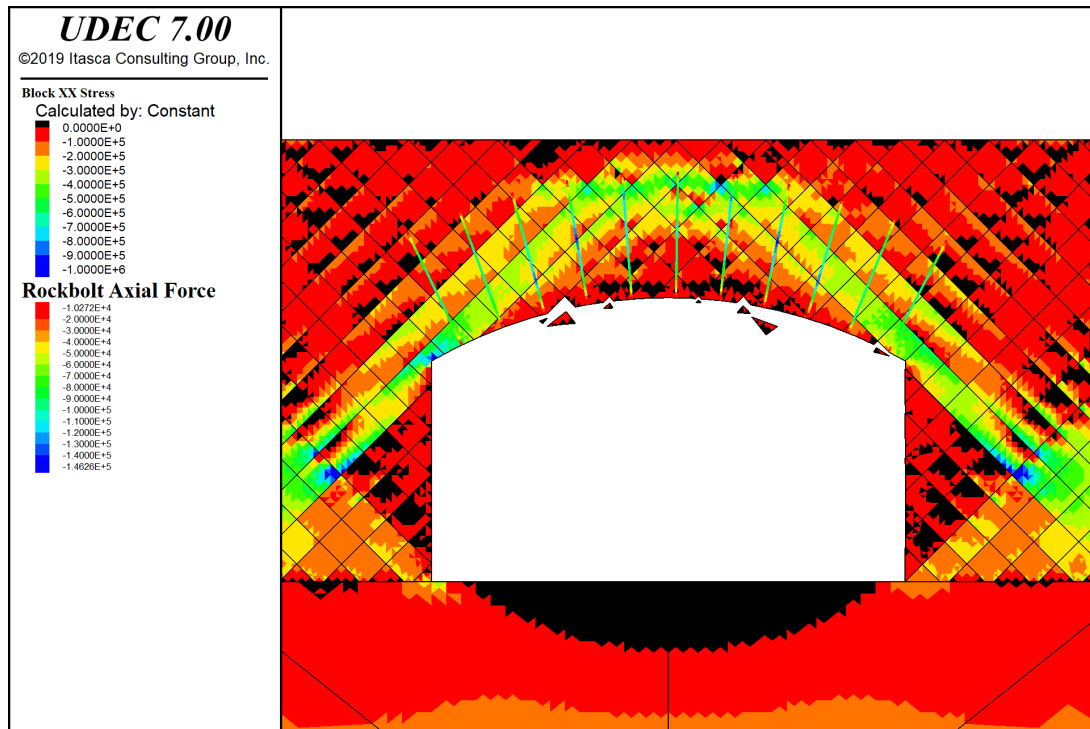
Exempel på utvecklade tryckspänningar vid numerisk analys av valvstabilitet med UDEC för ytlig tunnel.
